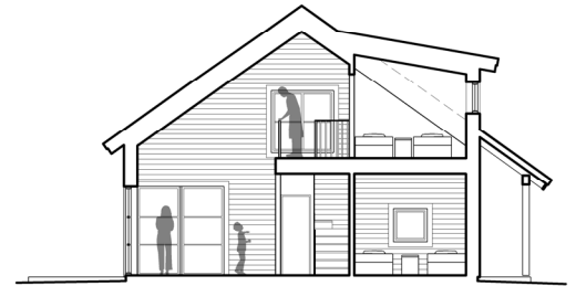
PRINCIPSNITT
